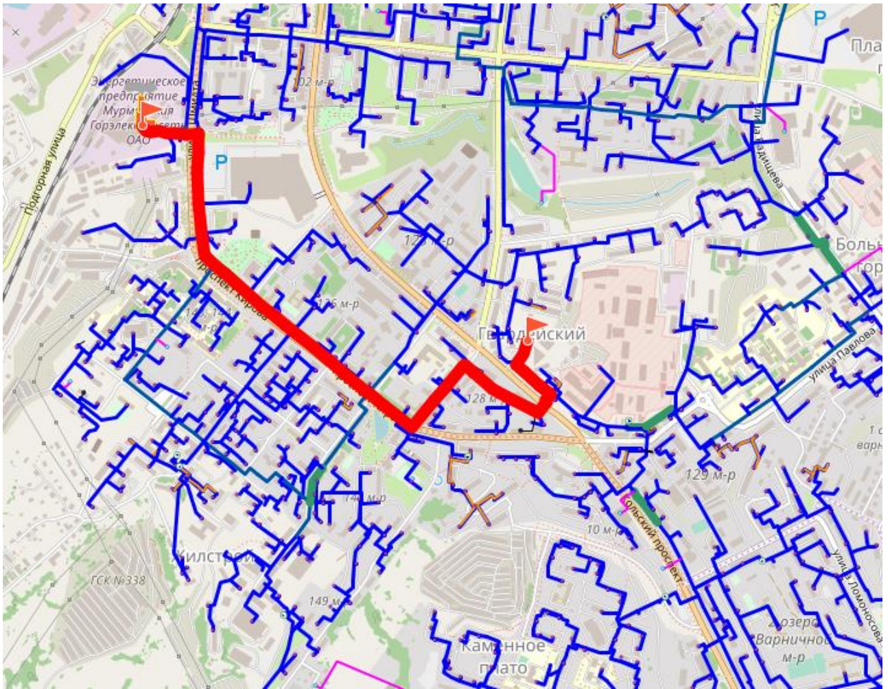
Рисунок 4.5 Путь для построения пьезометрического графика от Мурманской ТЭС до многоэтажной застройки
