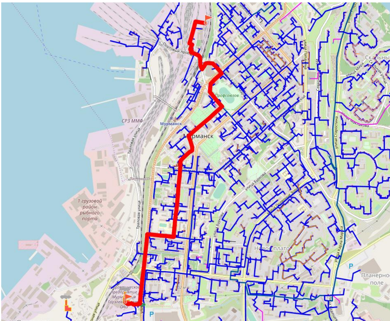
Рисунок 4.7 Путь для построения пьезометрического графика от Мурманской ТЭЦ до ОАО «РЖД»
