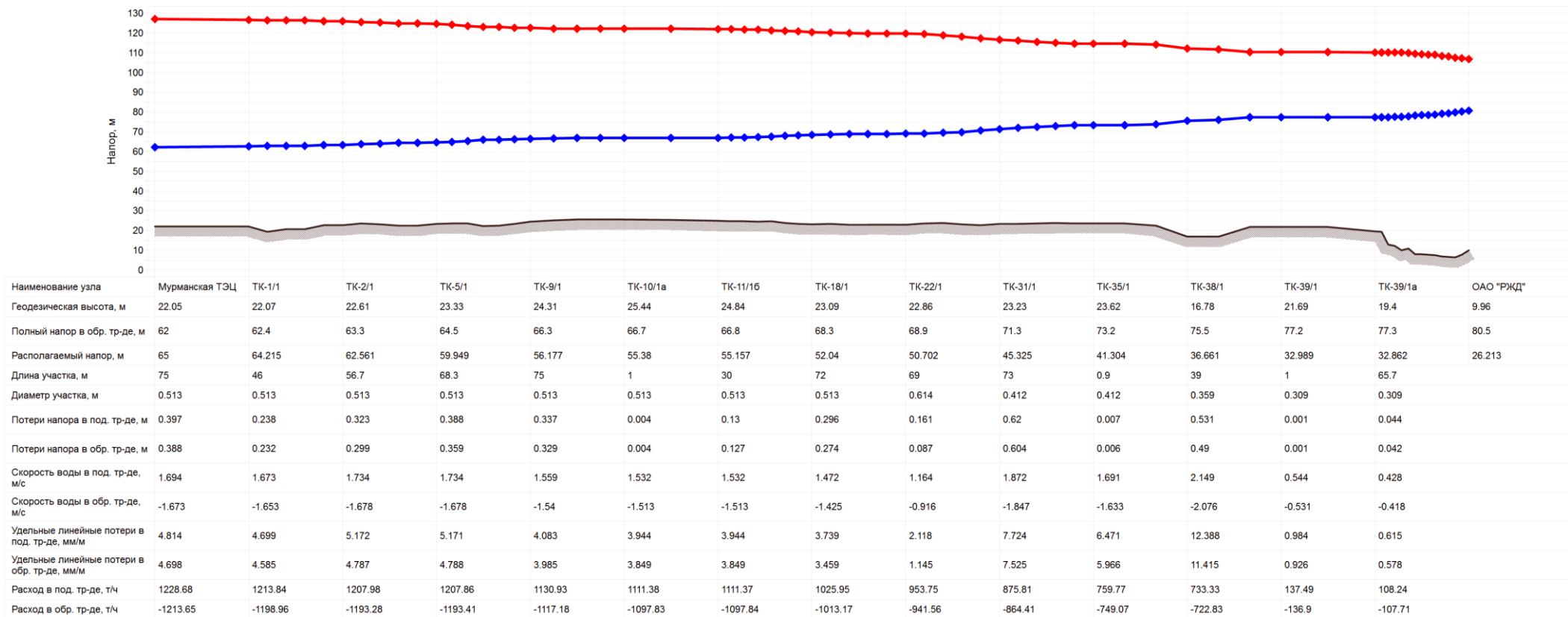
Рисунок 4.8 Пьезометрический график участка тепловой сети от Мурманской ТЭС до ОАО «РЖД»
