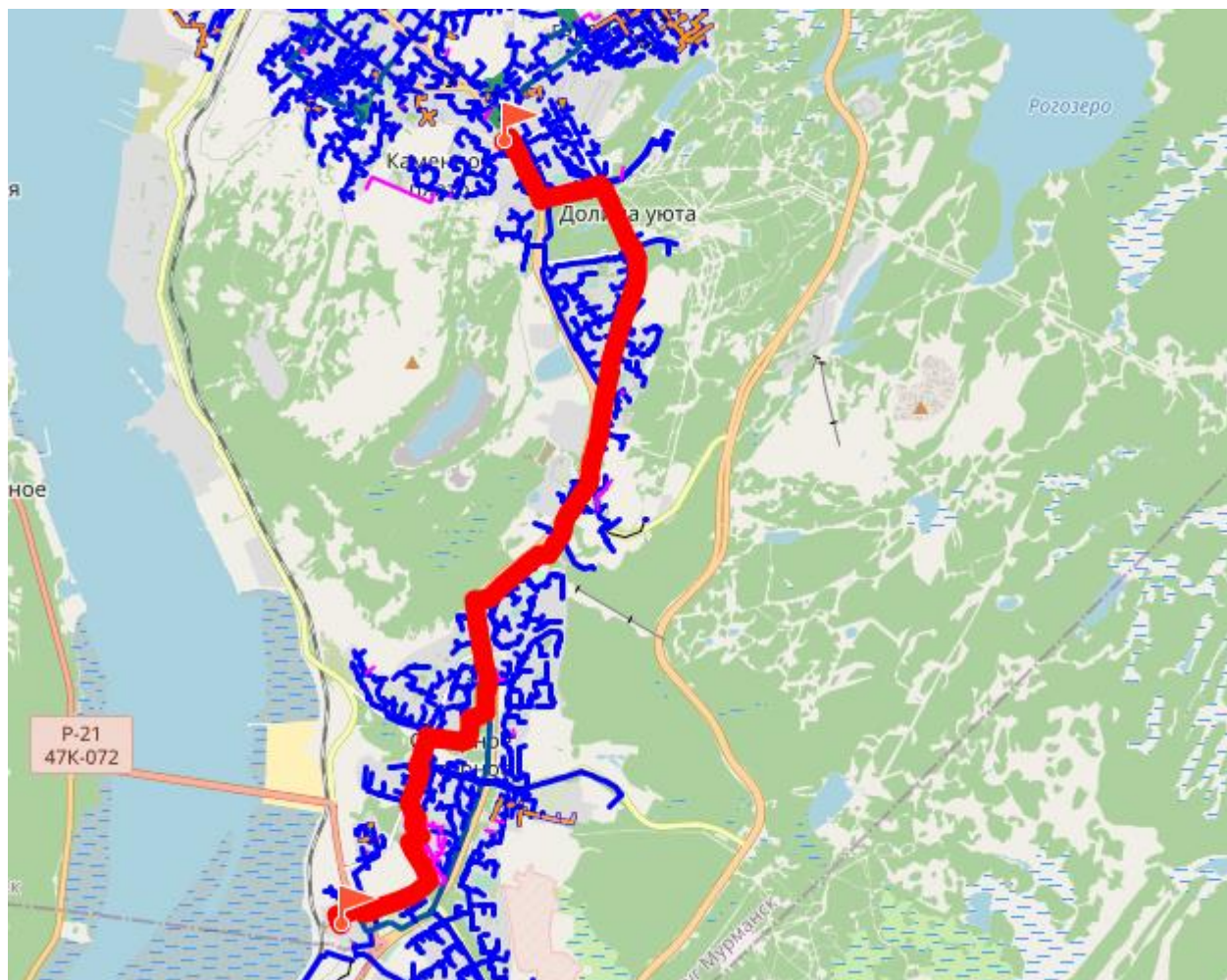
Рисунок 4.9 Путь для построения пьезометрического графика от Южной котельной до ООО «Аванта»
