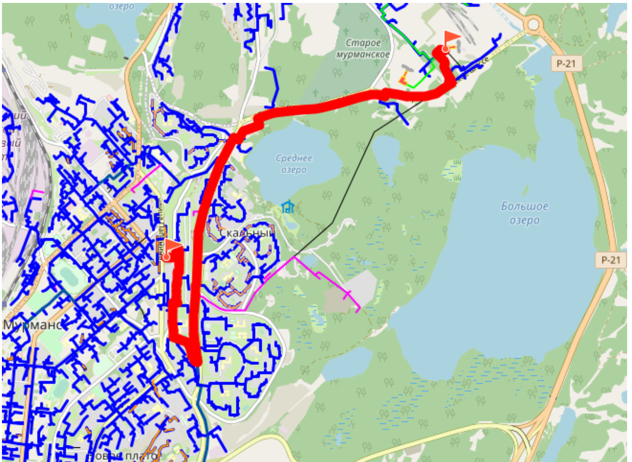
Рисунок 4.15 Путь для построения пьезометрического графика от Восточной котельной до перспективного потребителя многоэтажной жилой застройки
