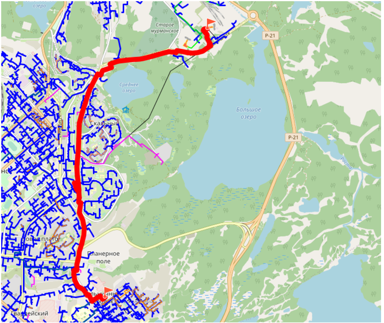
Рисунок 4.17 Путь для построения пьезометрического графика от Восточной котельной до застройки в Больничном городке
