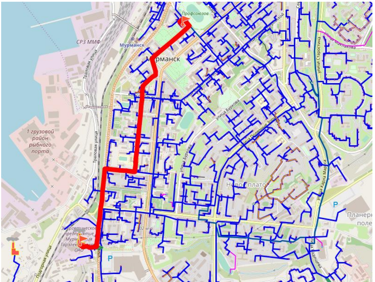
Рисунок 4.3 Путь для построения пьезометрического графика от Мурманской ТЭЦ до кинотеатра «Родина»
