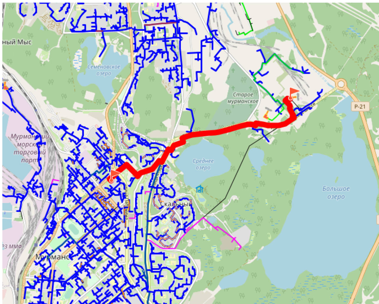
Рисунок 4.13 Путь для построения пьезометрического графика от Восточной котельной до перспективного потребителя многоэтажной жилой застройки
