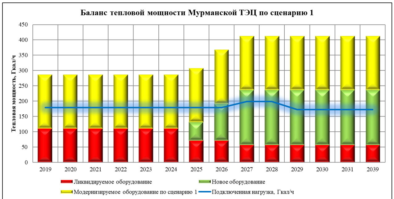
Рисунок 7.4 Баланс тепловой мощности Мурманской ТЭЦ на период актуализации Схемы теплоснабжения по сценарию 1 и 2
