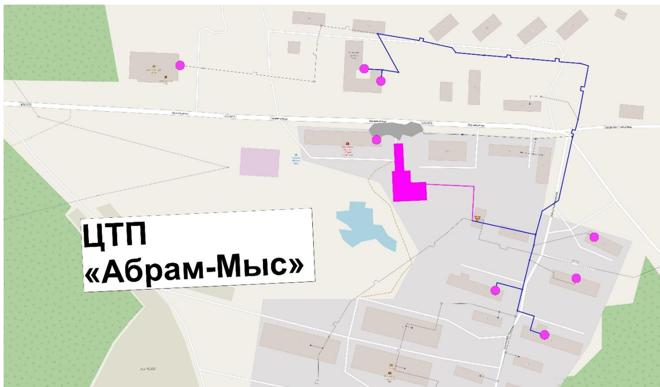
Рисунок 7.11 Расположение ЦТП №1
