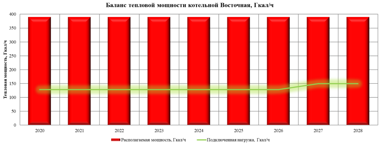
Рисунок 7.5 Баланс тепловой мощности Восточной котельной для Сценария 1 и Сценария 2 (до 2028)
