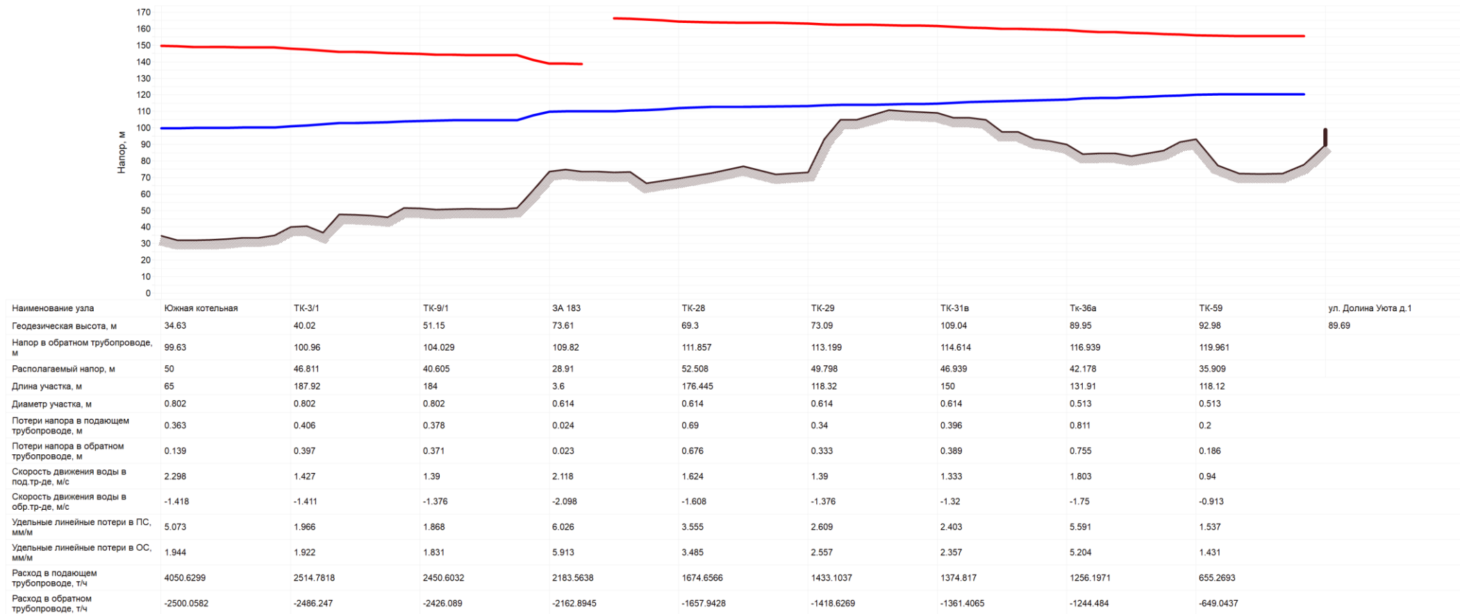
Рисунок 3.29 Существующий гидравлический режим тепловых сетей от Южной котельной
