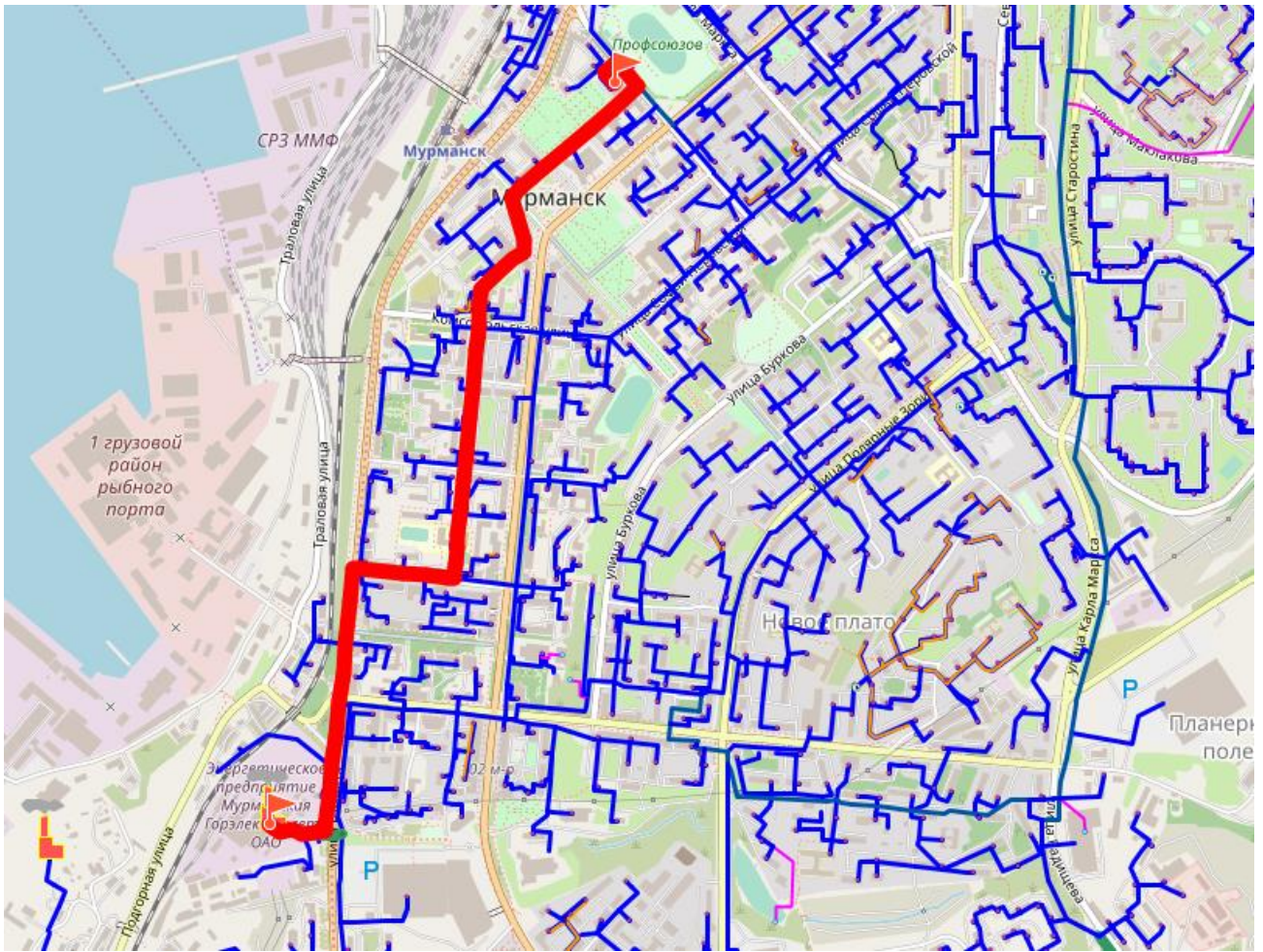
Рисунок 4.3 Путь для построения пьезометрического графика от Мурманской ТЭС до кинотеатра «Родина»
