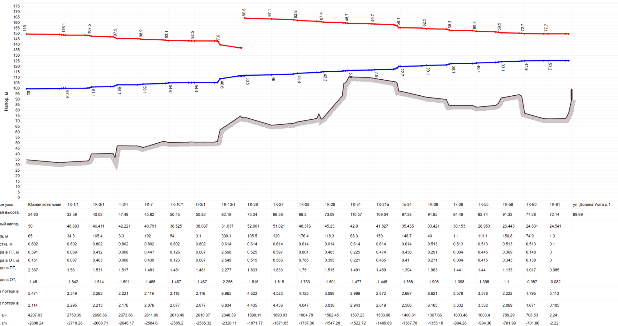
Рисунок 4.10 Пьезометрический график участка тепловой сети от Южной котельной до перспективного потребителя (Здание Российской учебно-спортивной базы, Долина Уюта,1)
