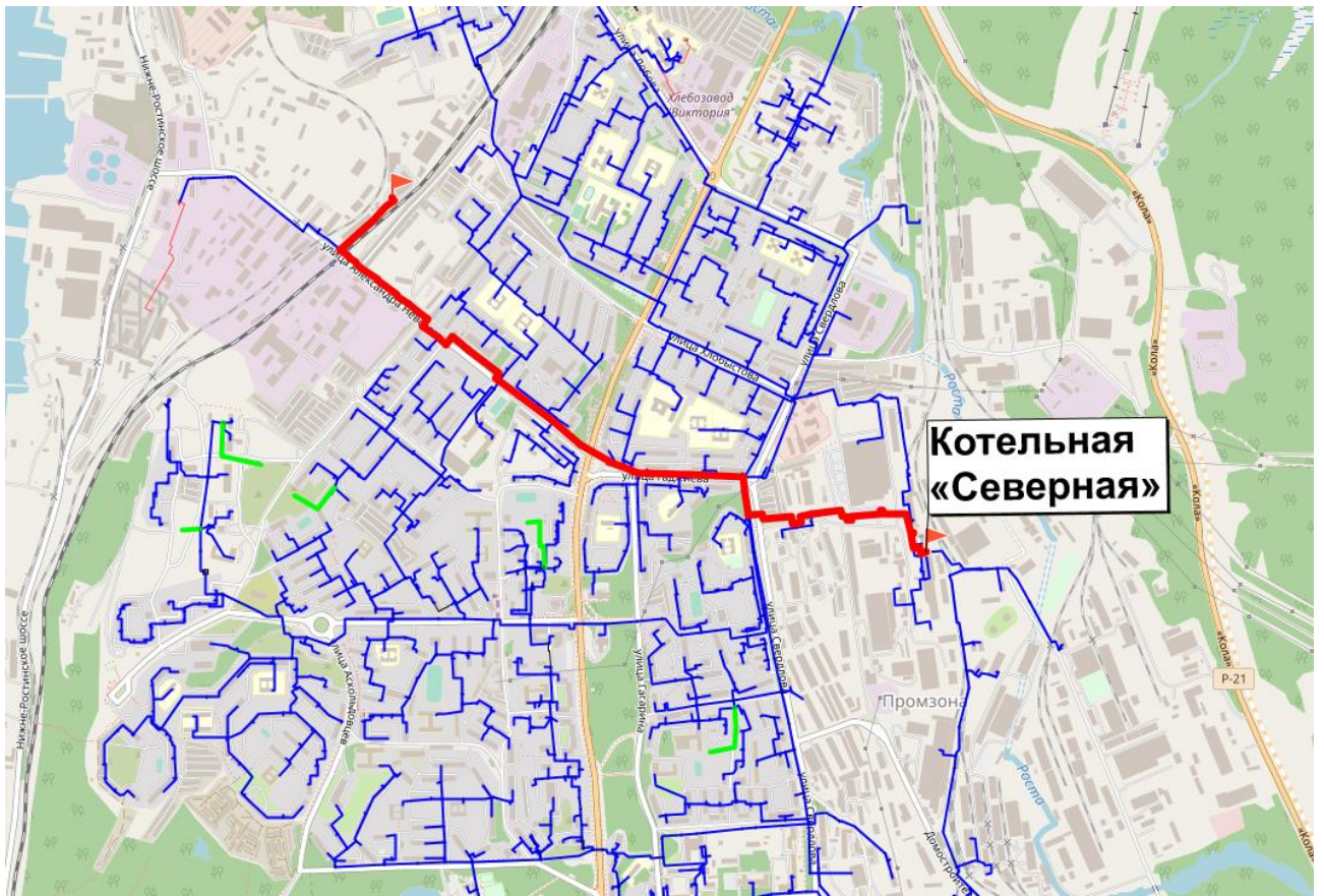
Рисунок 4.21 Путь для построения пьезометрического графика от котельной «Северная» до перспективного потребителя (АБК, ул.Александра Невского, д.59, к.1)
