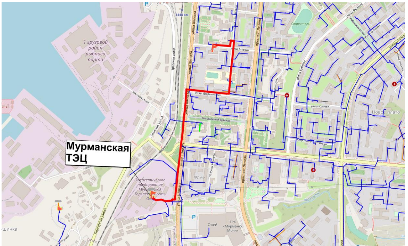
Рисунок 4.7 Путь для построения пьезометрического графика от Мурманской ТЭС до потребителя ул.Егорова, 6
